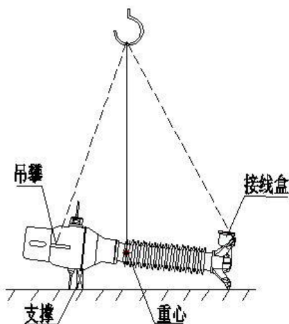
图 1 水平状态
