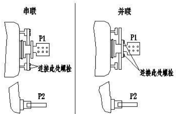
图 5 串并联换接方式 1
