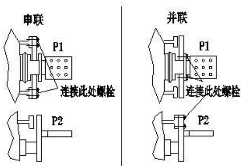
图 5 串并联换接方式 2
