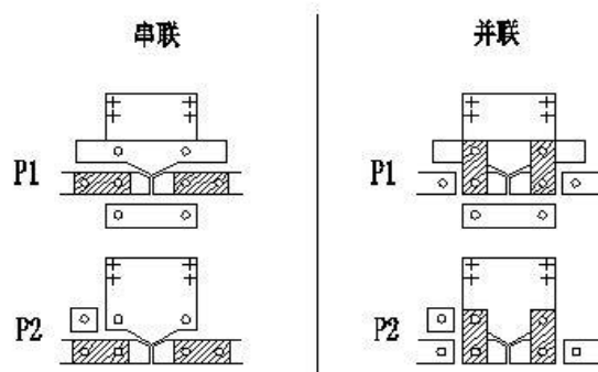
图 5 串并联换接方式 3
