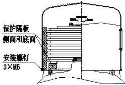
图 4 膨胀器保护隔板图
