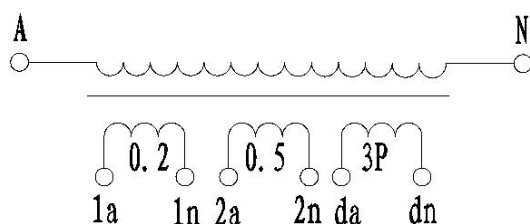
图 1 JDZXF9-35W 电压互感器原理图
