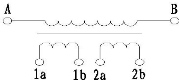
图 1 JDZ9-10 电压互感器原理图
