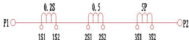
图 1 LZW-10 电流互感器原理图
